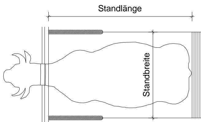
Abbildung 9: Vermessung der Standlänge und der Standbreite
