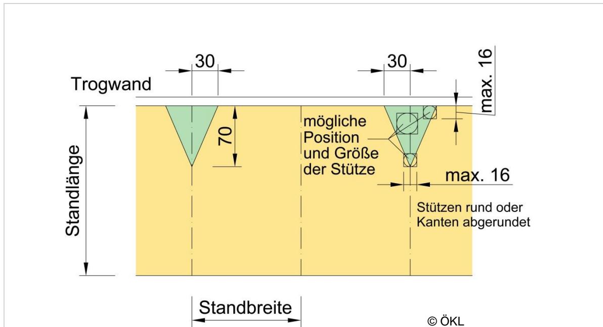
Abbildung 10: Beurteilung baulicher Elemente bei der Vermessung des Standes
