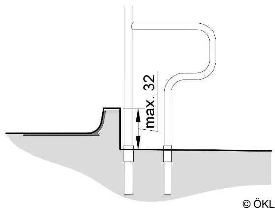
Abbildung 7: Maße zum massiven Barnsocket
